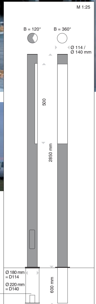
Lichtauslasswinkel B · angle of light outlet B
